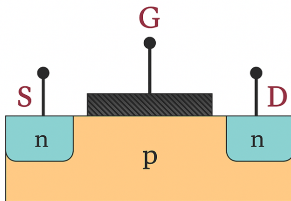
Figura 2.1: Estructura MOSFET de canal N [1]
